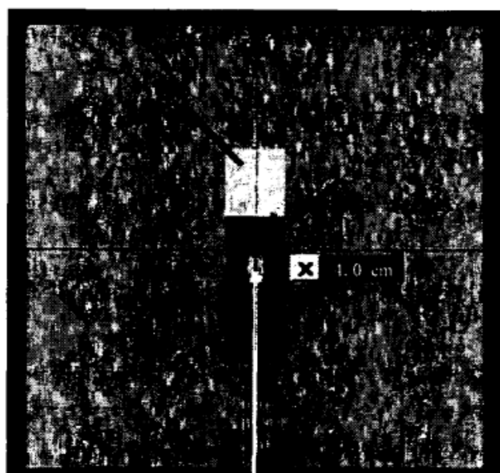
图 A.2 模拟多靶区冠状面
