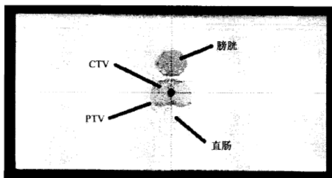
图 A.4 模拟前列腺肿瘤横断面
