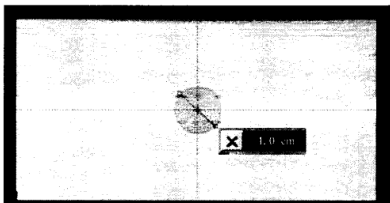
图 A.3 模拟多靶区横断面
