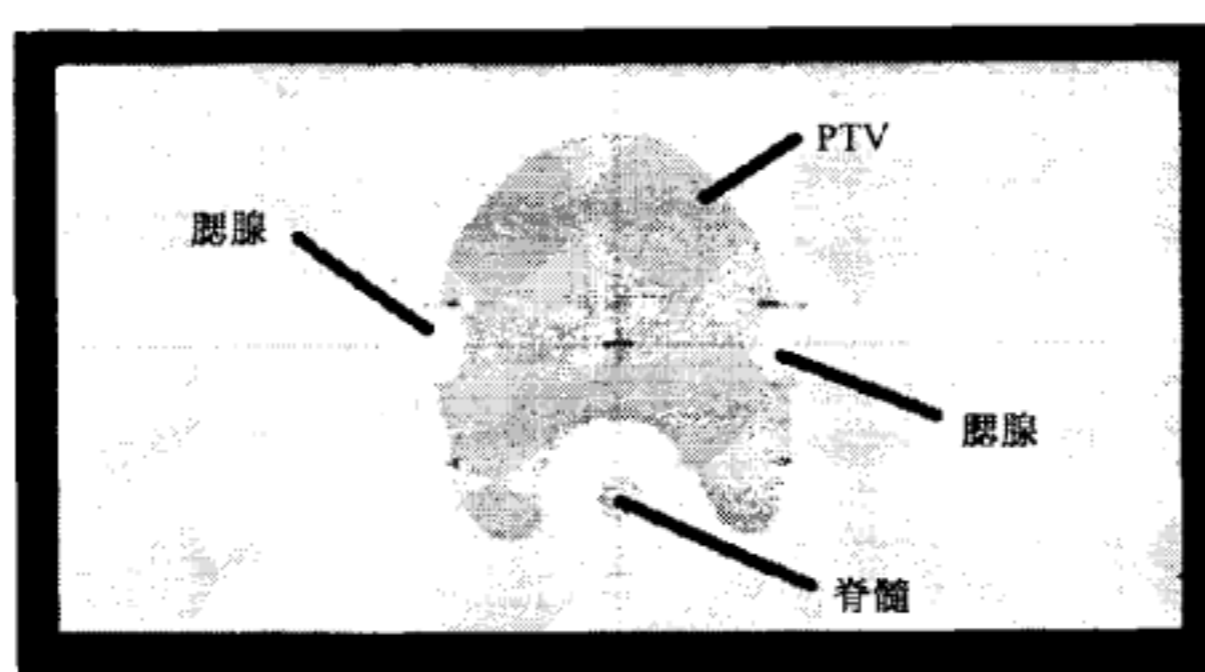
图 A.6 模拟头颈肿瘤横断面
