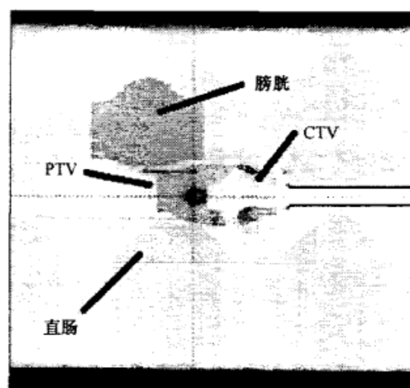
图 A.5 模拟前列腺肿瘤冠状面
