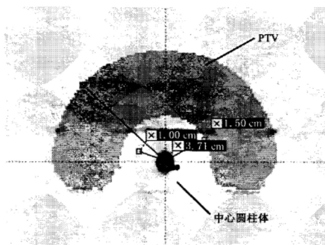
图 A.8 模拟 C 型靶区横断面
